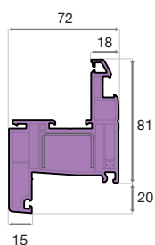
Profils des dormants
